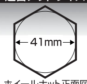
ホイールナット正面図
