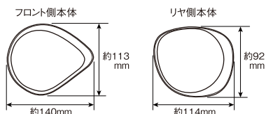
寸法図
