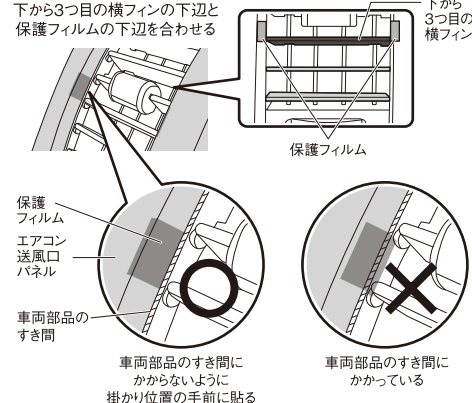
保護フィルム貼付箇所(2箇所) 横ツメ掛かり位置
