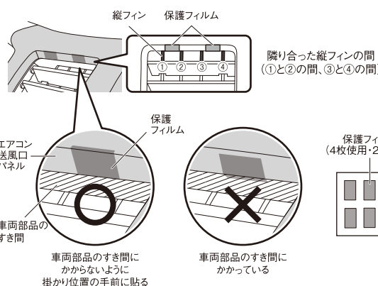
(図4) 保護フィルム貼付箇所(2箇所) 上ツメ掛かり位置
