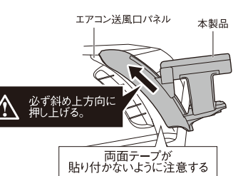
(図6) 【横から見た図】
