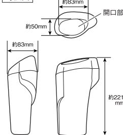
寸法図
