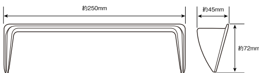
寸法図
